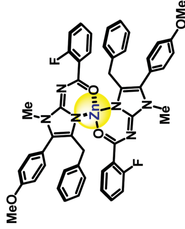
Zn(ZNA)_2
