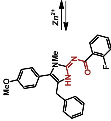
zinaamidole (ZNA)
