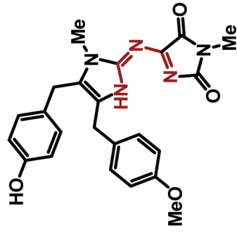
naamidine A
